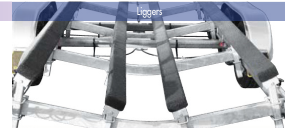
Verstelbaar achterbalk
